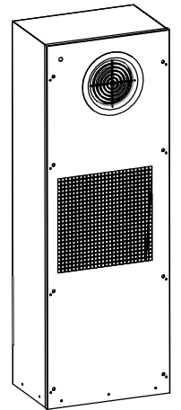
外形尺寸和开口尺寸 Dimensions and openings dimensions
